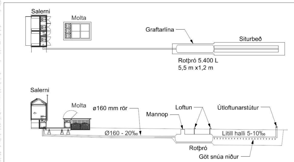
Skýringarmynd - Gestaskjól, salerni og rotþró. Mkv. 1:250
