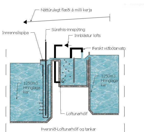
Mynd 17: Þversniðu af loftun á eldisvatni.
