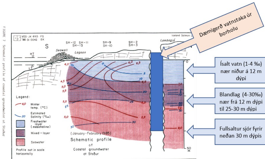
Mynd 41: Þversnið af vatnsgeymi í hrauninu.
